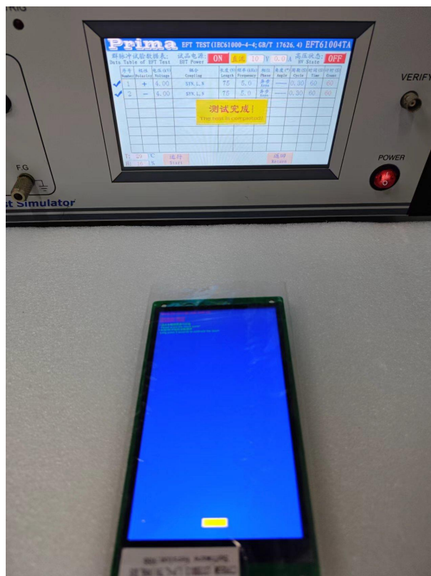
图 5-4 群脉冲测试图
