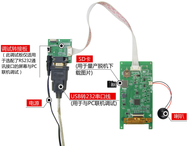
图 1-3 调试工具图
