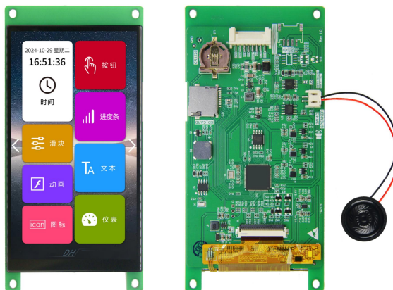
图 1-1 5.0 寸电容触摸参考图
