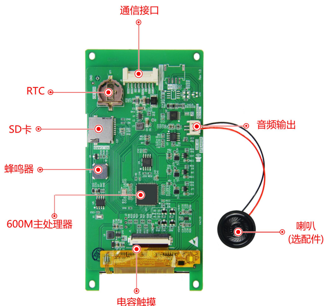
图 1-2 硬件配置图
